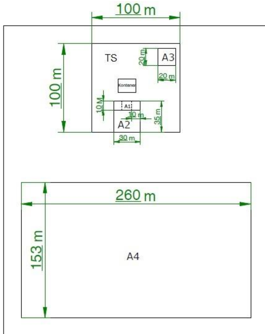
Rys. 1 Układ wolier adaptacyjnych dla drobia
